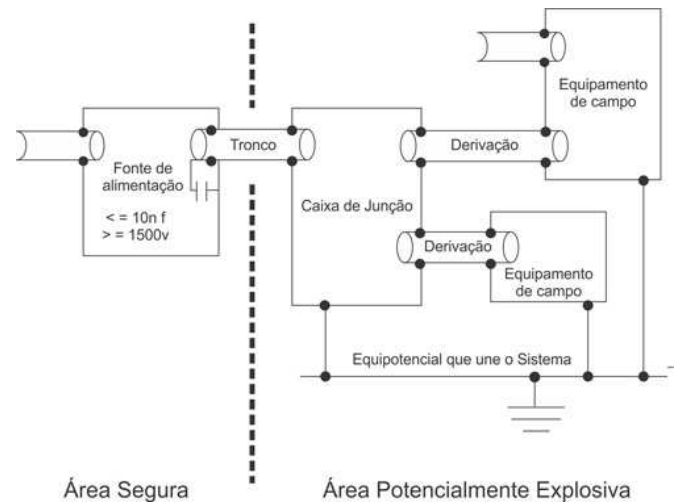
Figura 10 – Aterramento capacitivo.
