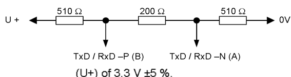
Figura 5 – Terminador RS485-IS.
