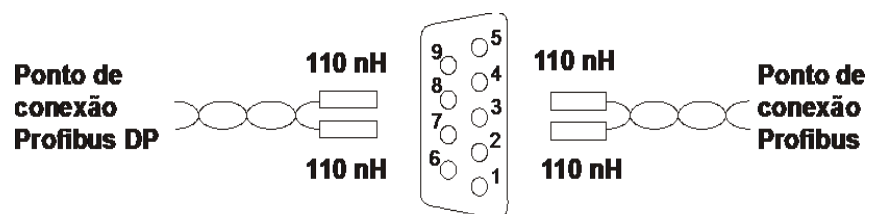
Figura 3 – Ligação de conectores e indutores na rede Profibus-DP.
