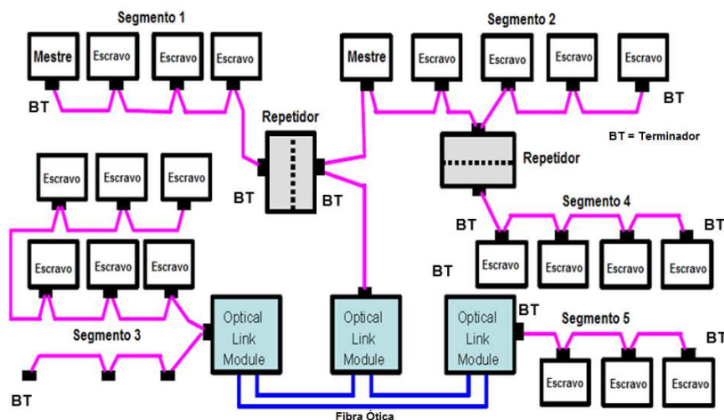
Figura 4 – Repetidores, terminadores e link óticos.
