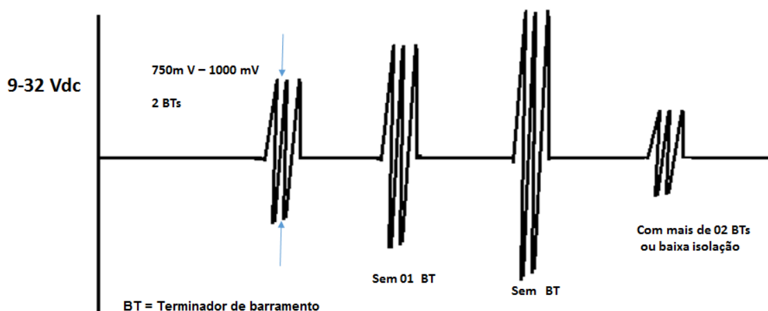
Figura 8 – Formas de onda típicas do Profibus-PA, de acordo com a terminação.
