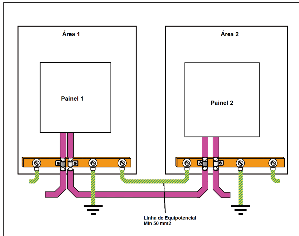
Figura 15 – Sistema de aterramento com diferentes áreas em Profibus-DP.
