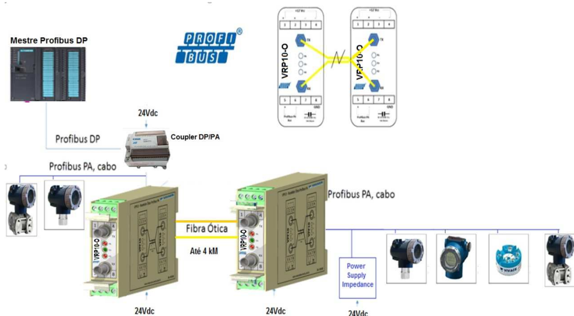
Figura 11– Repetidor ótico Profibus-PA.
