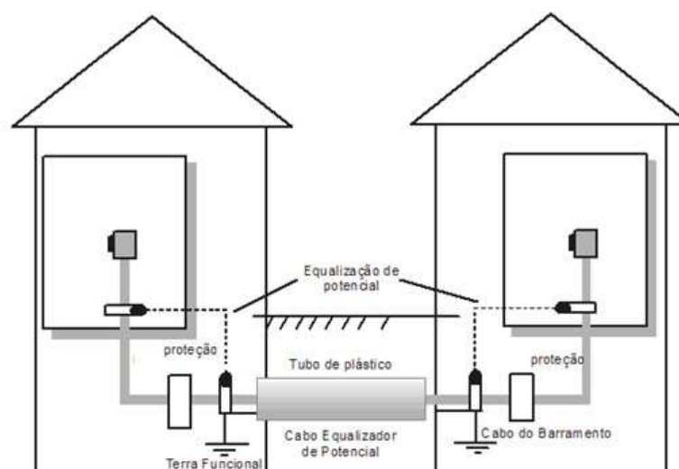
Figura 16 - Detalhe de cabeamento em áreas distintas com potenciais de terras equalizados.
