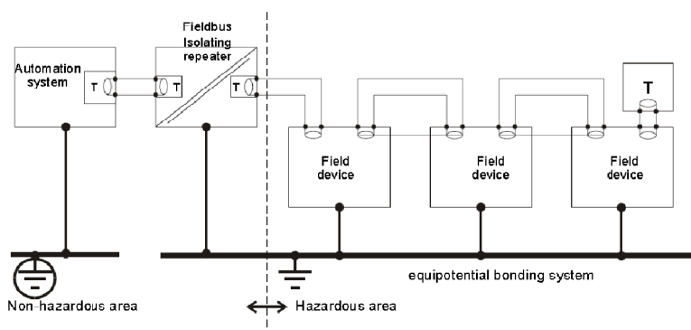
Figura 6 – Shield e aterramento no RS485-IS.
