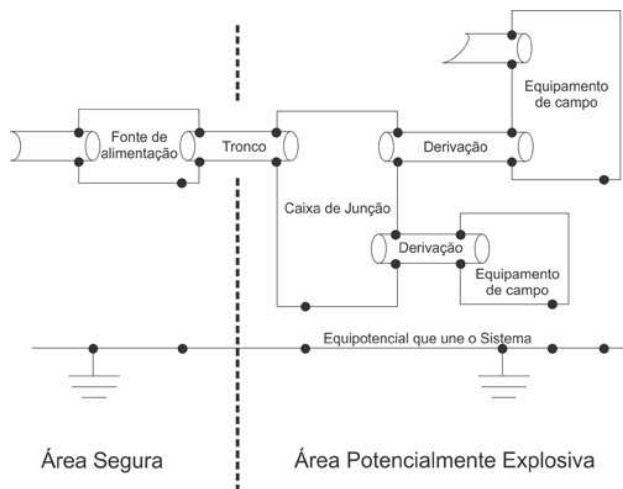
Figura 9 – Combinação ideal de shield e aterramento.
