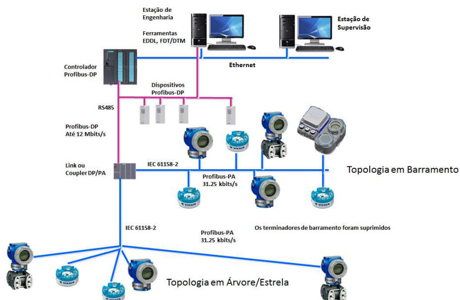
Figura 12 – Profibus-PA: IEC 61158-2 - Topologias em barramento e árvore/estrela.
