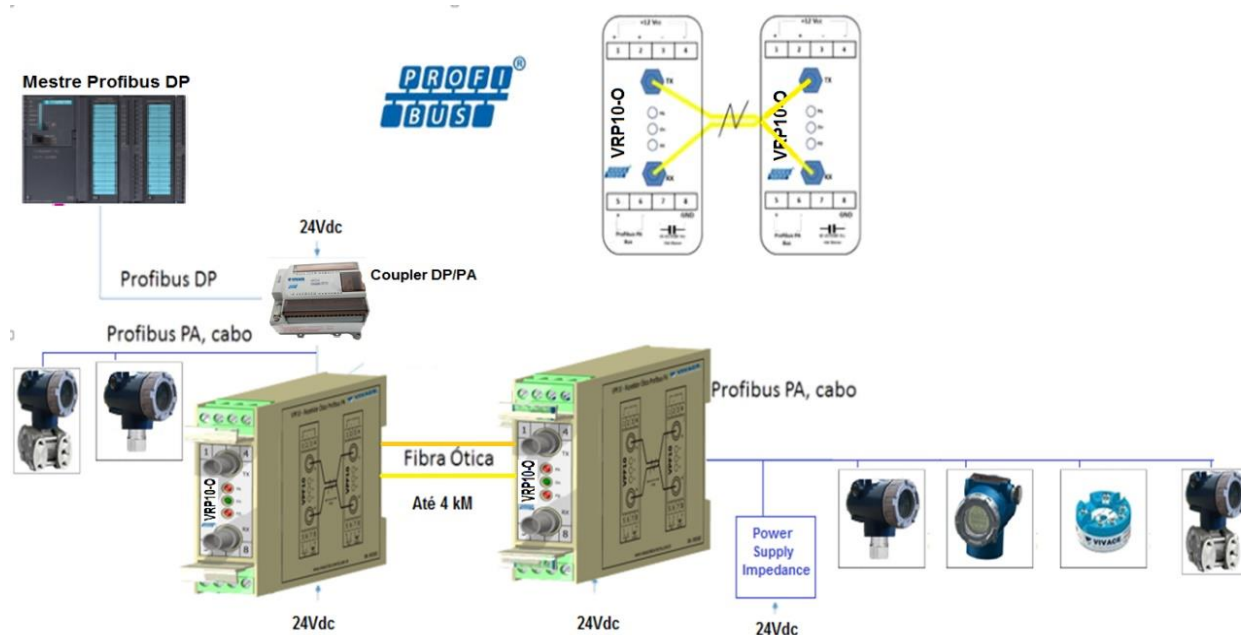
Figura 11– Aplicação típica do VRP10-O, repetidor óptico Profibus-PA.
