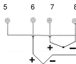
Conexão termopar ou mV diferencial
