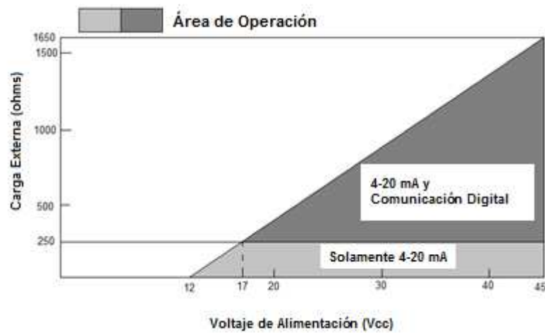
Figura 3.4 – Caída de voltaje del VTT10-PH.
