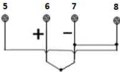
Figura 2.8 - Conexión termopar o mV.
