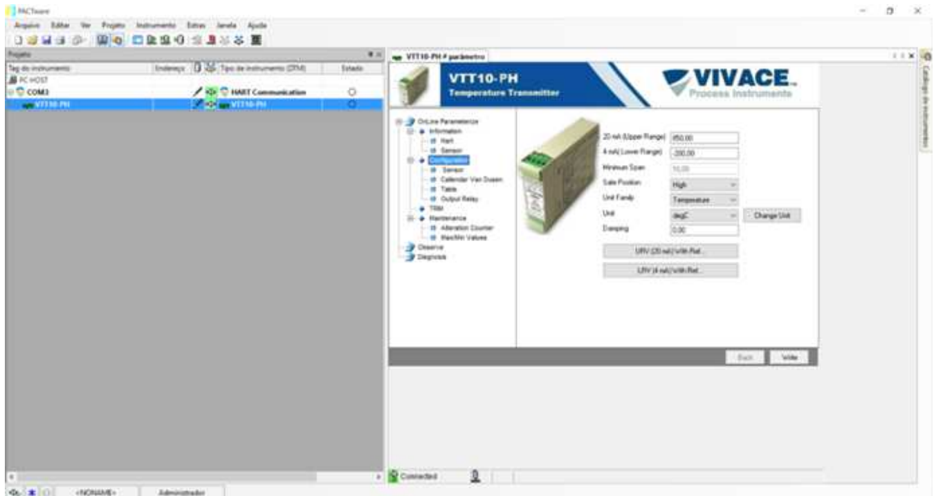
Figura 3.7 – Pantalla de configuración del rango de trabajo del VTT10-PH en PACTware.
