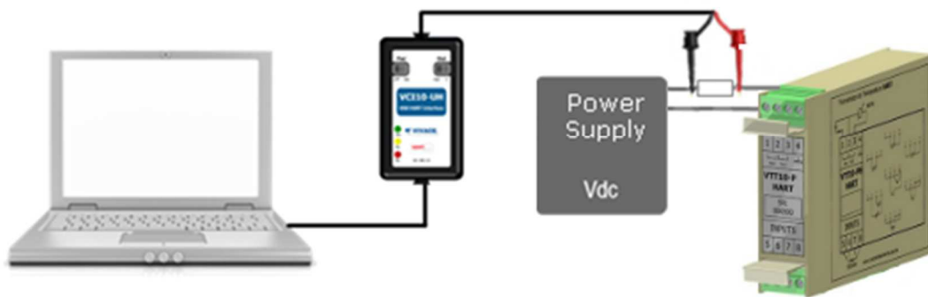
Figura 3.1 - Esquema de conexión de la interfaz VCI10-UH al VTT10-PH con alimentación externa.
