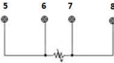
Figura 2.6 - Conexión RTD o resistivo a 4 hilos.
