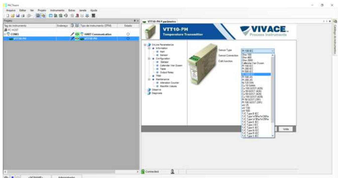
Figura 3.8 – Pantalla de configuración del sensor de VTT10-PH en PACTware.
