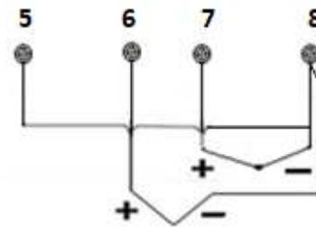
Figura 2.9 - Conexión termopar o mV diferencial, máximo, mínimo y backup.
