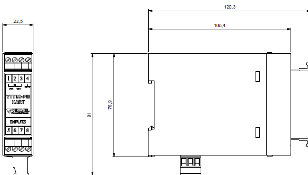
Figura 2.2 - Diseño dimensional del VTT10-PH con salida discreta.
