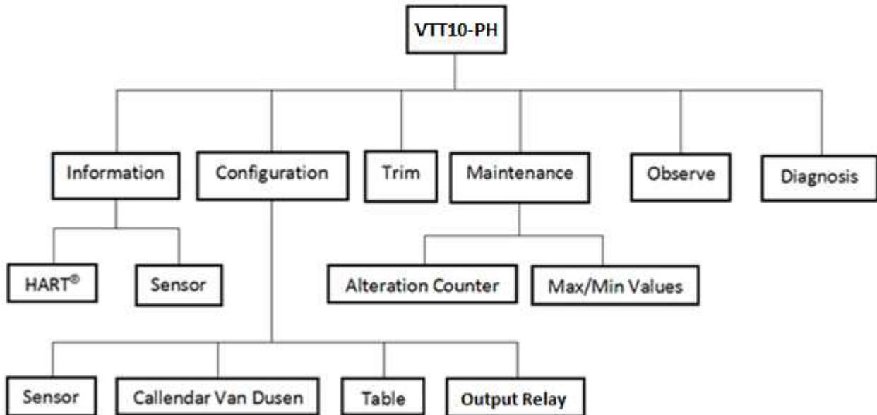
Figura 3.5 – Árbol de programación del VTT10-PH.
