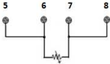
Figura 2.4 - Conexión RTD o resistivo a 2 hilos.
