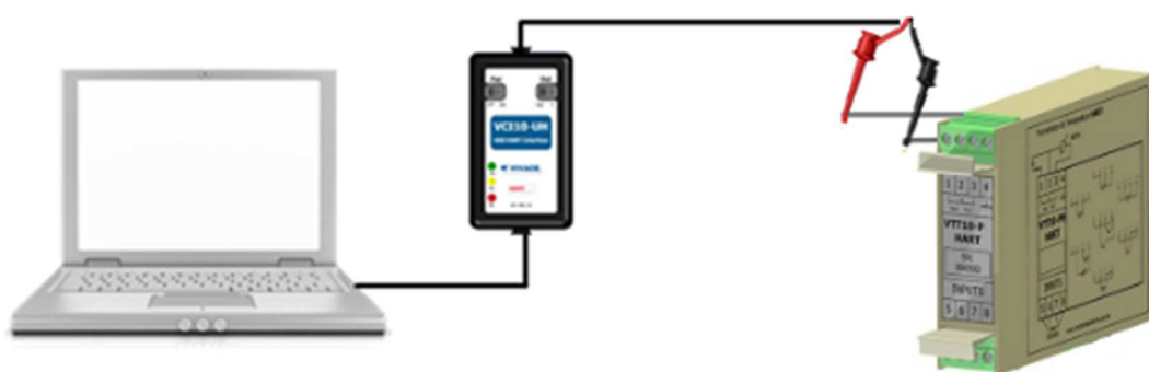
Figura 3.2 - Esquema de conexión de la interfaz VCI10-UH alimentando el VTT10-PH.
