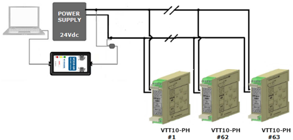
Figura 3.3 – Esquema de conexión de la interfaz al VTT10-PH en configuración multidrop.
