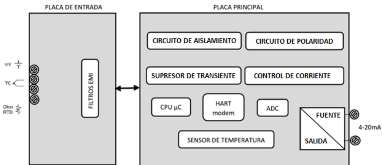
Figura 1.1 - Diagrama de bloques del VTT10-PH.
