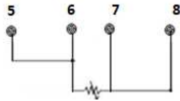
Figura 2.5 - Conexión RTD o resistivo a 3 hilos.
