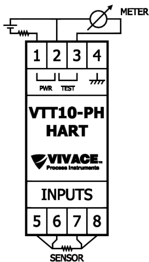
Figura 2.3 – Conexiones de los terminales del VTT10-PH.
