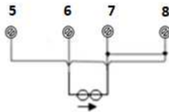
Figura 2.10 - Conexión entrada corriente 4 - 20 mA.
