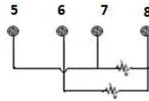
Figura 2.7 - Conexión RTD o resistivo diferencial, máximo, mínimo y backup.
