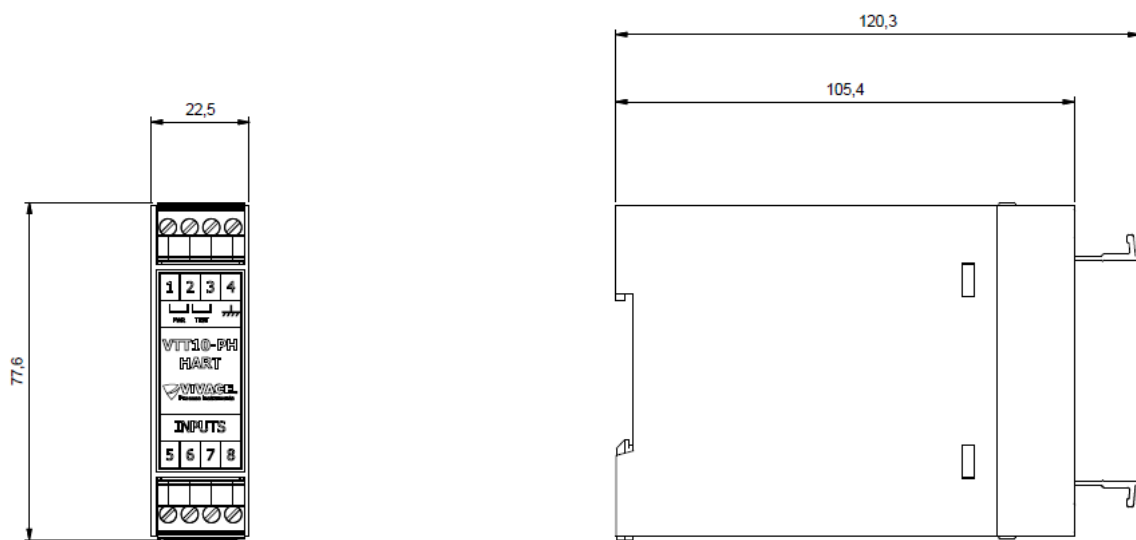
Figura 2.1 – Diseño dimensional y esquema de montaje del VTT10-PH.
